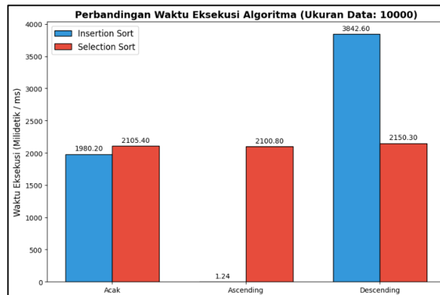
Gambar 1. Contoh Penyajian Gambar Grafik Perbandingan Waktu Eksekusi N = 10000
