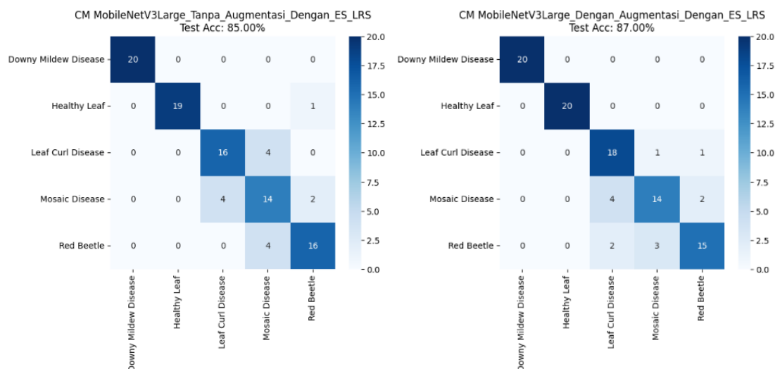
Gambar 6. Confusion Matrix MobileNetV3-Large (Dataset Orisinal) dan (Augmentasi Data)
