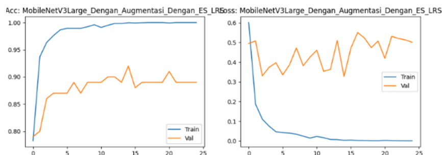
Gambar 5. Grafik Acc-Loss MobileNetV3-Large (Dataset Orisinal) dan (Augmentasi Data)
