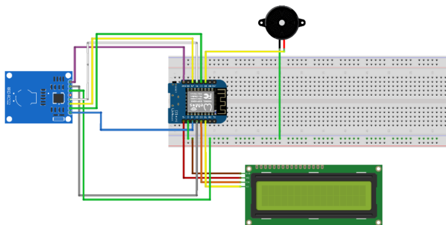
Gambar 3. Diagram Rangkaian Sistem Absensi Berbasis RFID dan IoT.
