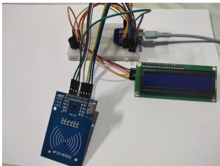
Gambar 4. Prototipe Sistem Absensi Cerdas Berbasis RFID dan IoT.
