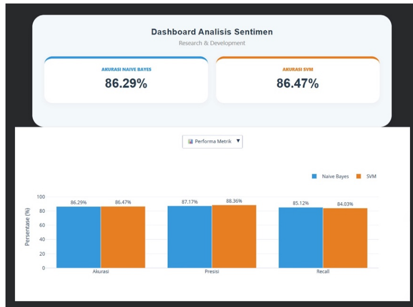
Gambar 1. Dashboard Analisis Sentimen Grafik Batang.
