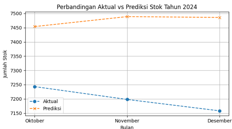
Gambar 4. Grafik Prediksi Stok 3 bulan kedepan 2024.
