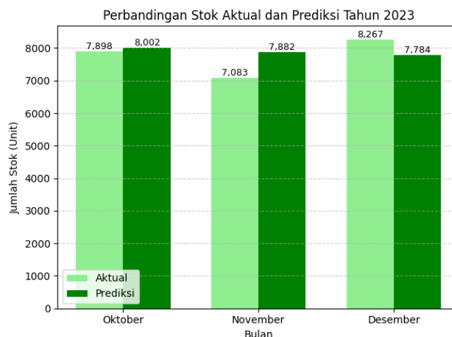
Gambar 9. Grafik Perbandingan Stok 2023.
