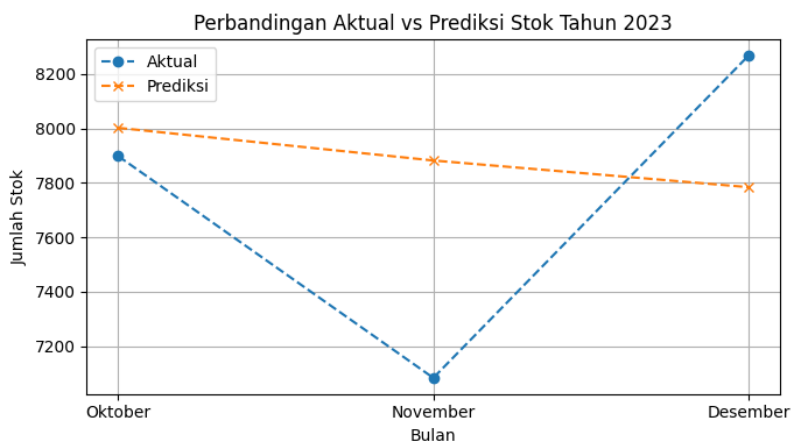
Gambar 3. Grafik Prediksi Stok 3 bulan kedepan 2023.
