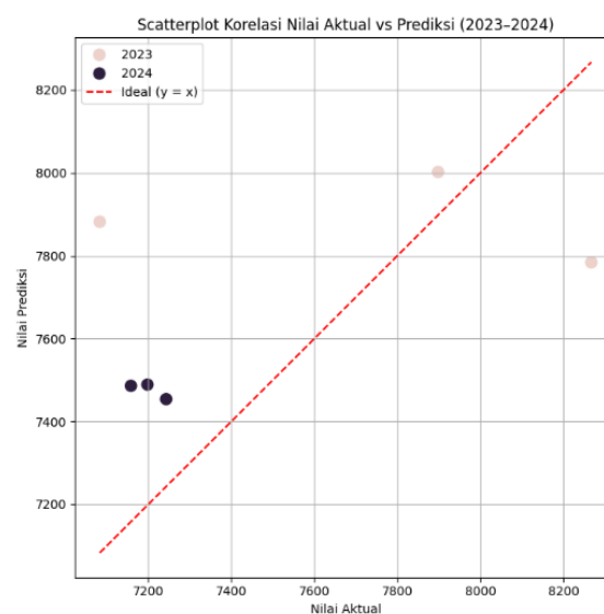
Gambar 12. Korelasi Prediksi Stok
