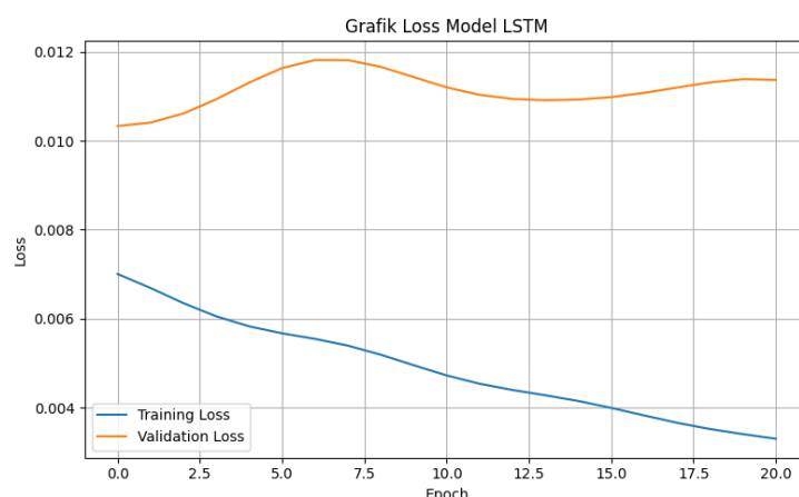
Gambar 5. Grafik Loss Pendapatan.
