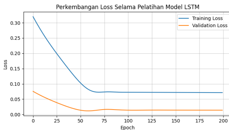
Gambar 6. Grafik Loss Stok..
